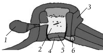
Four de fusion de Timna
